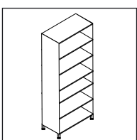
Стеллаж МЛ-900 ширина 80,1 глубина 45 высота 226,6
