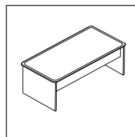
Стол рабочий МЛ-38М ширина 88 глубина 57,4 высота 46,6
