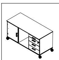
Тумба М-56Д ширина 138 глубина 58,8 высота 71,6
