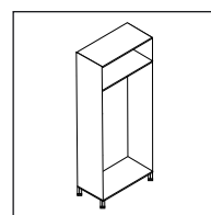
Стеллаж М-700С ширина 80,1 глубина 60 высота 190,4
