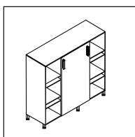
Стеллаж М-207 ширина 149,6 глубина 46,7 высота 141,8
