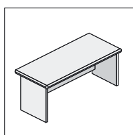
Стол рабочий NL201 длина 180 ширина 85 высота 75
