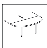
Сектор стола со стойкой К-374 длина 141,8 ширина 60 высота 76
