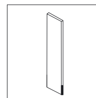
Стенка боковая стеллажа К-401 длина 38,8 ширина 1,8 высота 180,4
