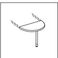
Сектор стола со стойкой К-372 длина 31 ширина 70 высота 76
