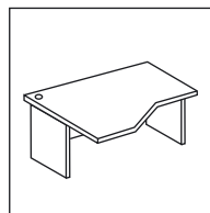
Стол письменный К-323Л/П длина 136 ширина 100/70/45 высота 76
