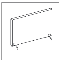
Перегородка К-630 ширина 156 высота 718 толщина 112,6
