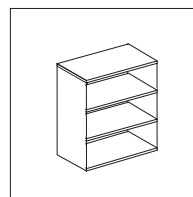
Стеллаж низкий К-20 ширина 80,6 глубина 41,6 высота 117,6
