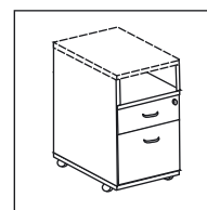
Тумба приставная с 2-мя ящиками К-521Т длина 44,4 ширина 45 высота 73,2
