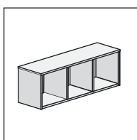
Полка навесная PПН ширина 111 глубина 32 высота 37
