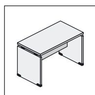
Стол приставной ПСП длина 100 ширина 60 высота 68
