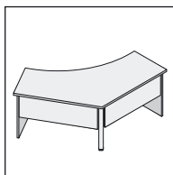
Стол рабочий ПСР16/ ПСР16У длина 160 ширина 80/60 высота 75
