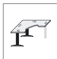
Стол рабочий л/п 25572/25573 длина 120/140 ширина 140/120 высота 71,5
