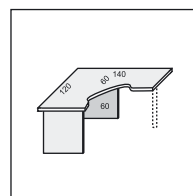
Стол рабочий л/п 25172/25173 длина 120/140 ширина 140/120 высота 71,5
